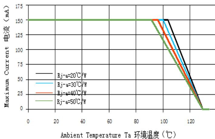
Thermal design 电流与环境温度曲线关系
